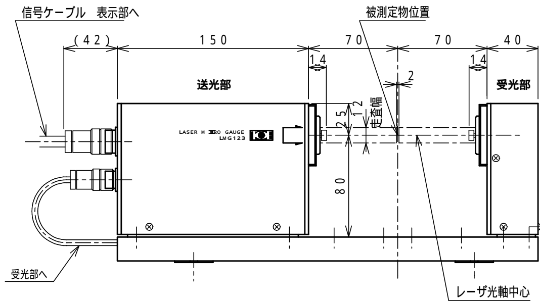
LMG 123 センサ部
