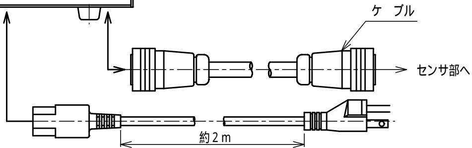
露点計 DPHシリーズ A型 表示部
