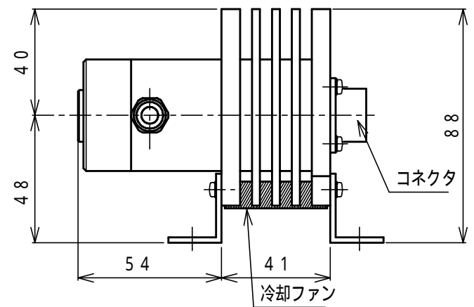
露点計 DPH - 203 センサ部
